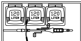
INNENRAUM
