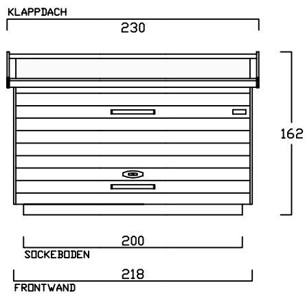
INNENMASS
