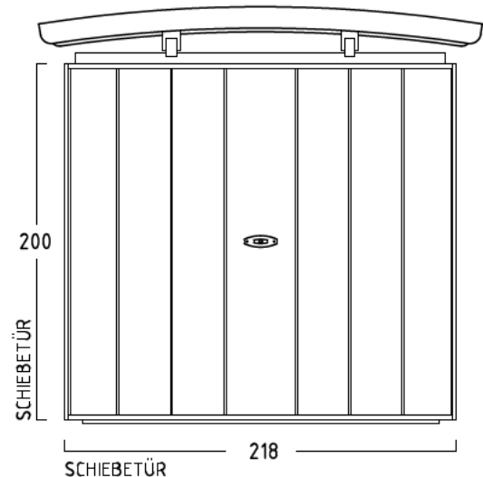
ANSICHT: SCHIEBETÜRFRONT OHNE VORBAU
