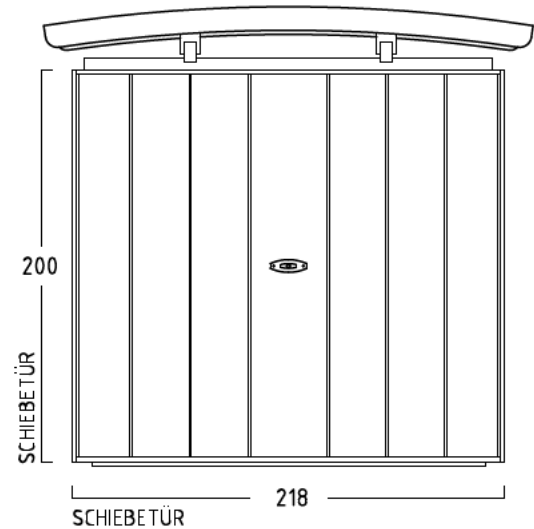
ANSICHT: SCHIEBETÜRFRONT OHNE VORBAU
